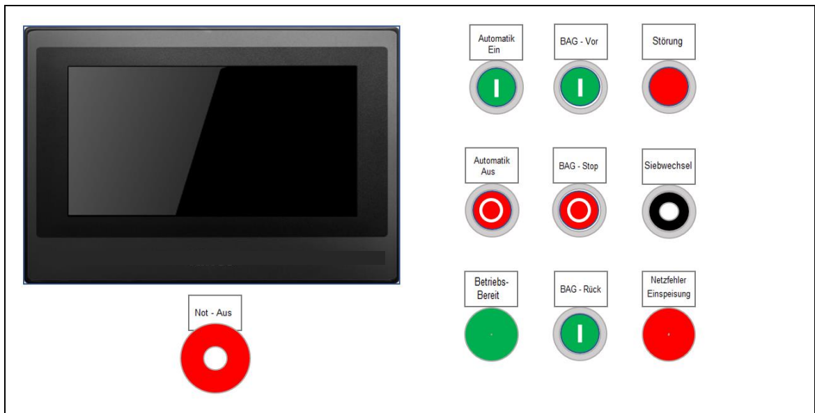
Abb. 4-3: Bedienanzeigen
