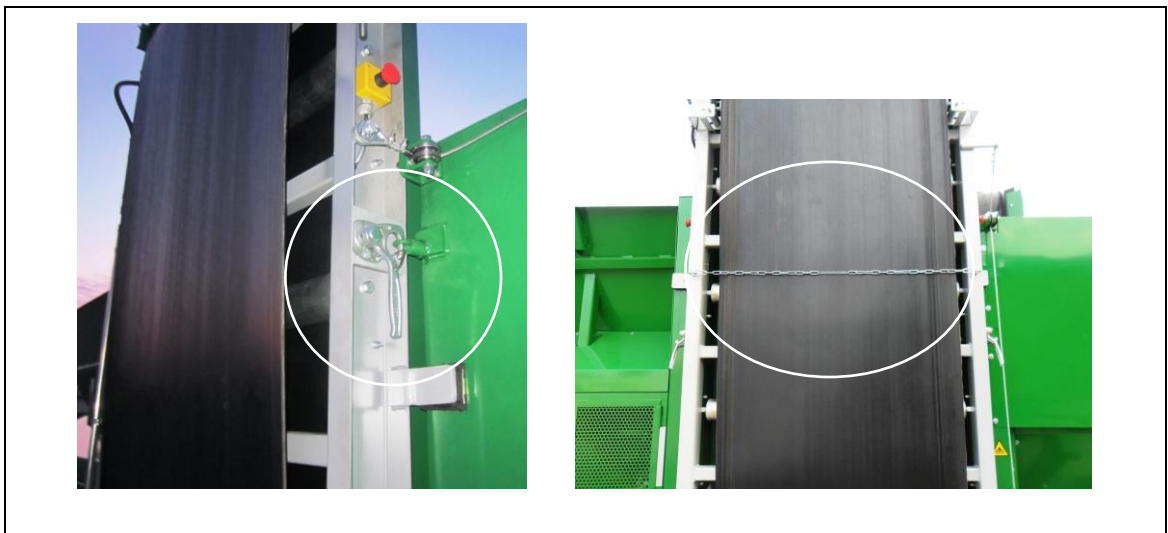
Abb. 7-2: Transportsicherung Feinfraktion
