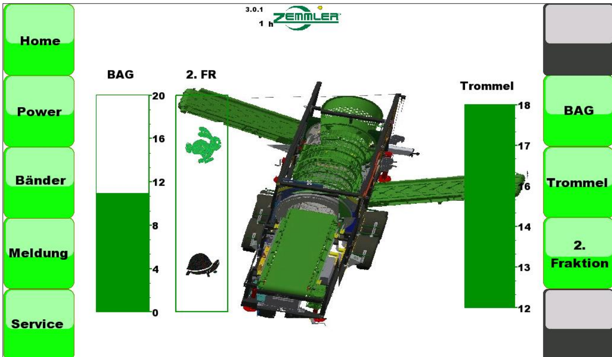
Abbildung 5 – Bänder-Bildschirm
