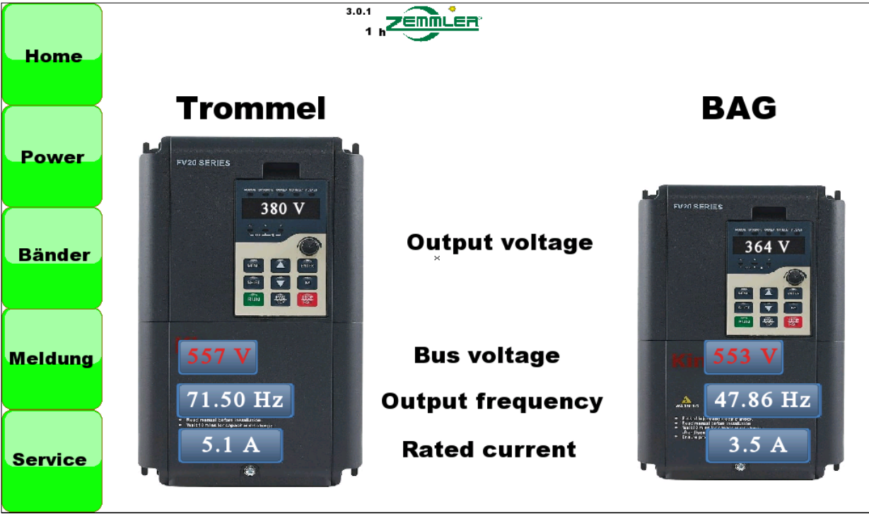
Abbildung 4 – Power-Bildschirm
