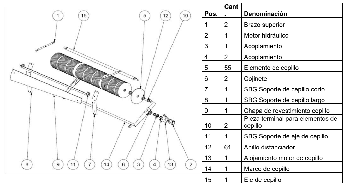
Fig. 11-5: Montaje y fijación del elemento de cepillo
