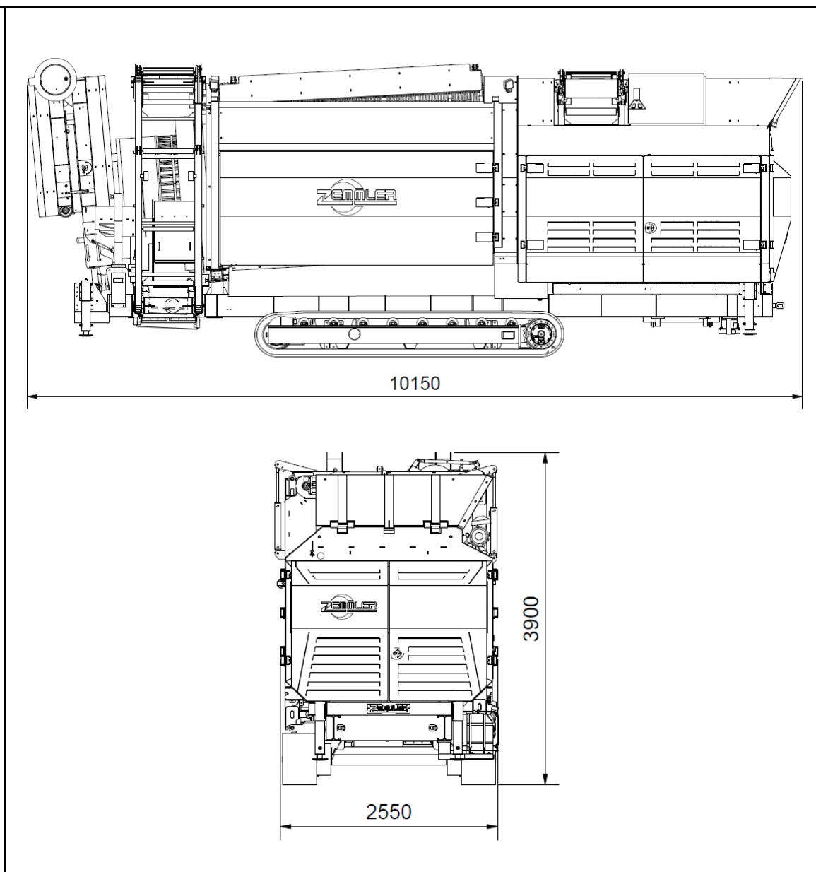
Fig. 12-3: Planta completa tren de rodaje de oruga (opción) Posición de trabajo con opción: cinta de fracción media y de fracción gruesa prolongada
