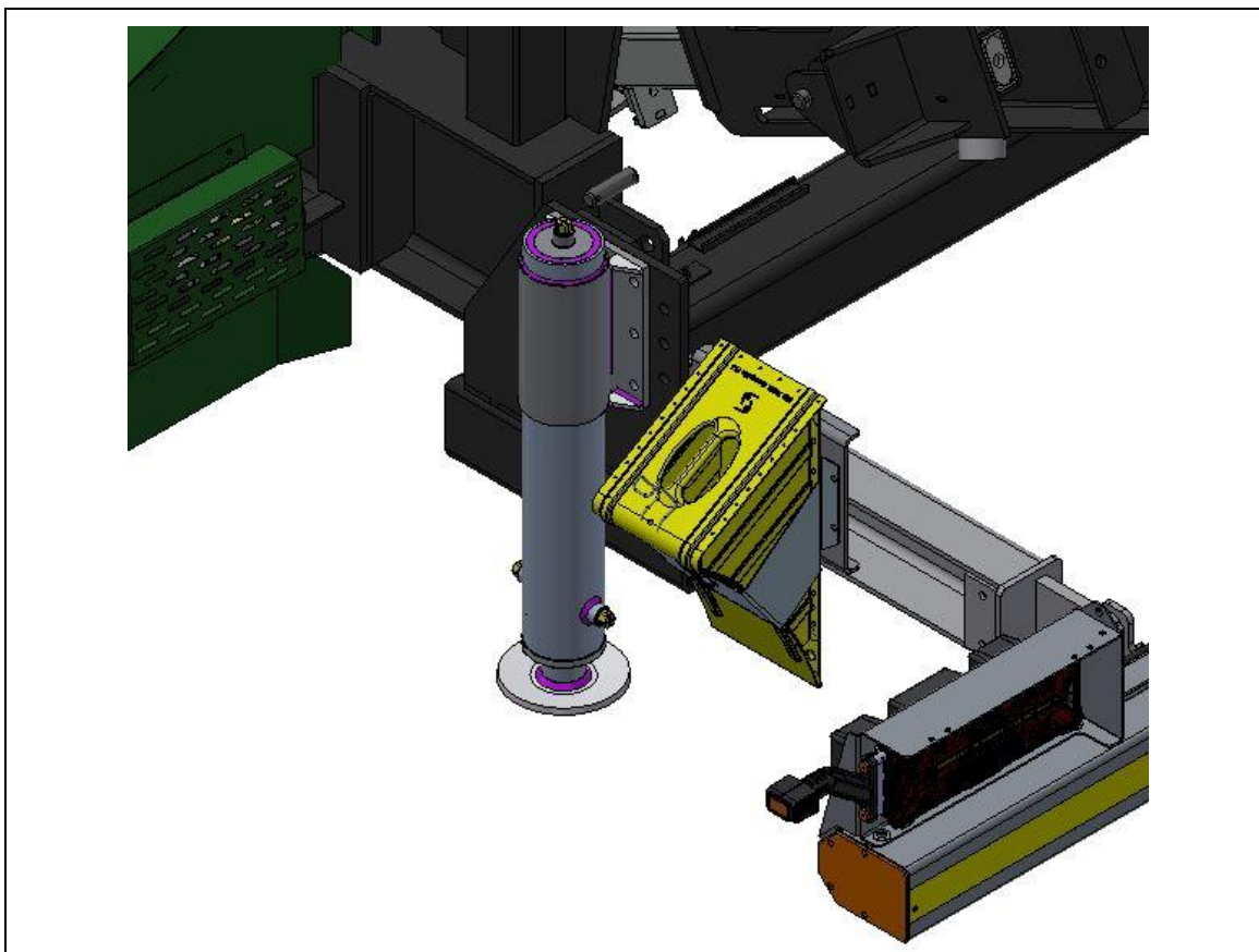
Fig. 7-2: Apoyos hidráulicos traseros
