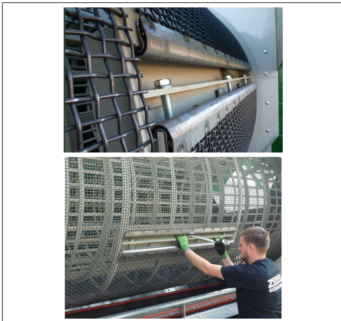
Fig. 11-3: Estación de tensado para el forro de cribado
