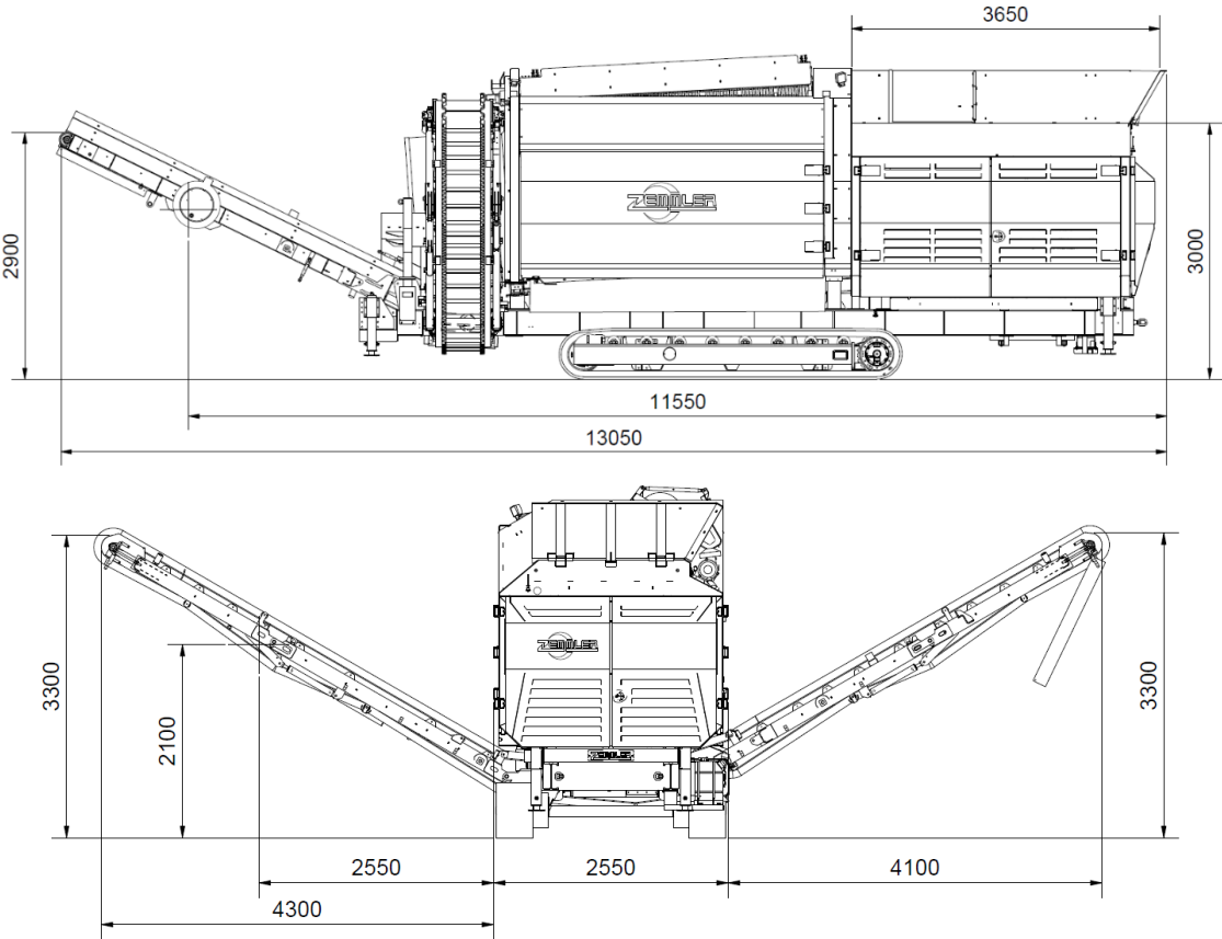
Fig. 12-4: Planta completa tren de rodaje de oruga (opción) Posición de trabajo con opción: cinta de fracción media y de fracción gruesa prolongada
