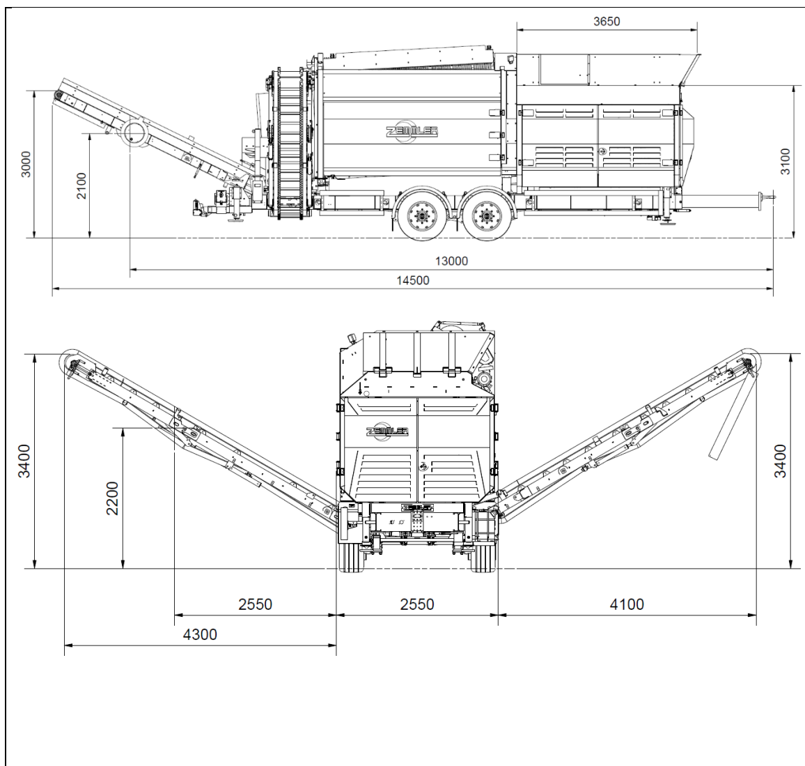
Fig. 12-2: Planta completa Posición de trabajo con opción: cinta de fracción media y de fracción gruesa prolongada
