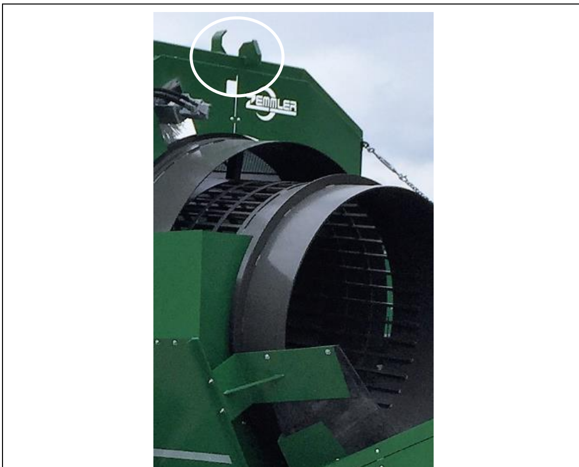
Fig. 7-6: Seguro de transporte de la fracción media prolongada
