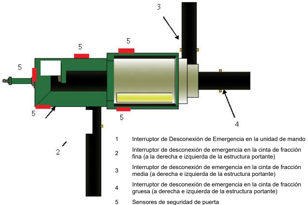
Fig. 3-1: Ubicación de los dispositivos de seguridad
