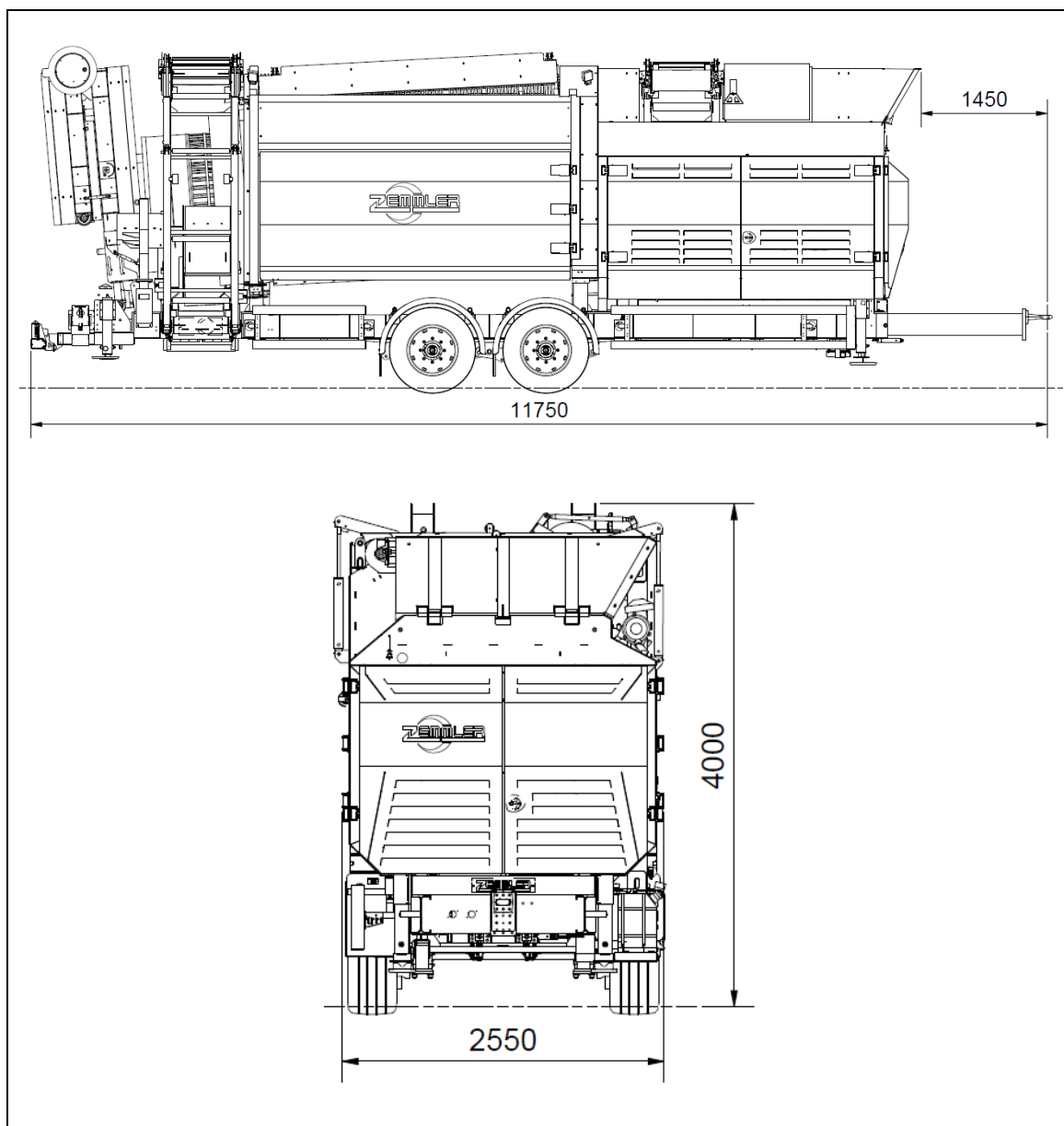
Fig. 12-1: Planta completa Posición de transporte con opción: cinta de fracción media y de fracción gruesa prolongada
