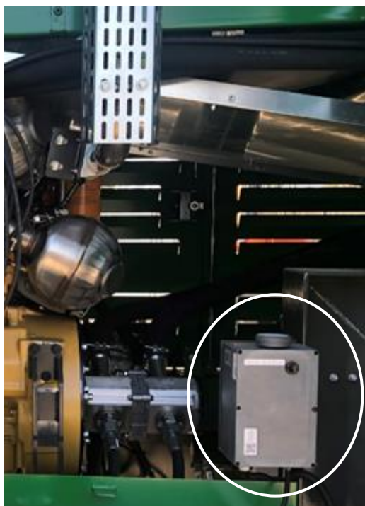
Fig. 11-7: Unidad de control de ventilador reversible en el compartimento interior de motor
