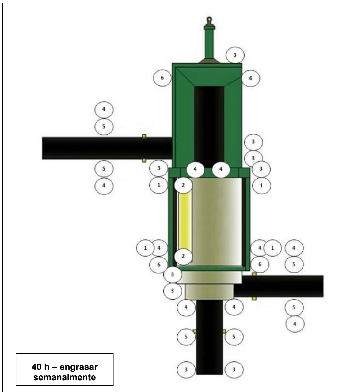
Fig. 11-4: Situación de los puntos de engrase
