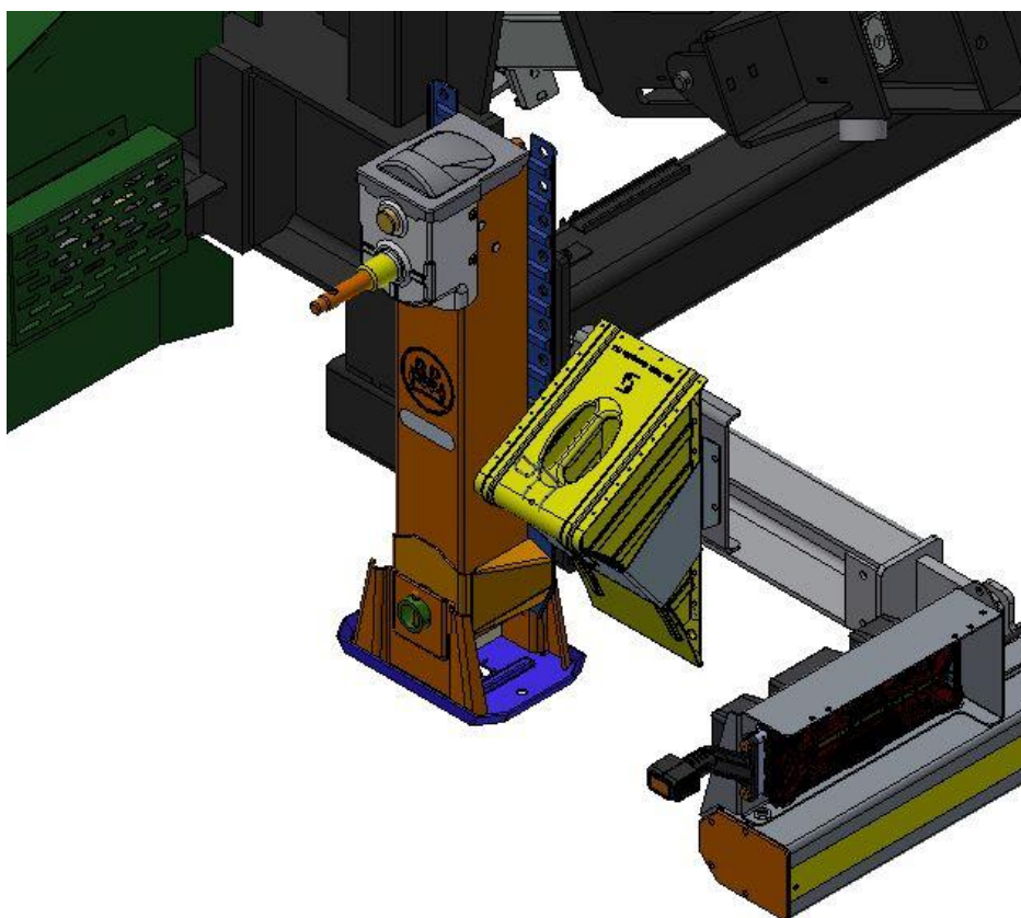
Fig. 7-1: Dispositivos de apoyo traseros
