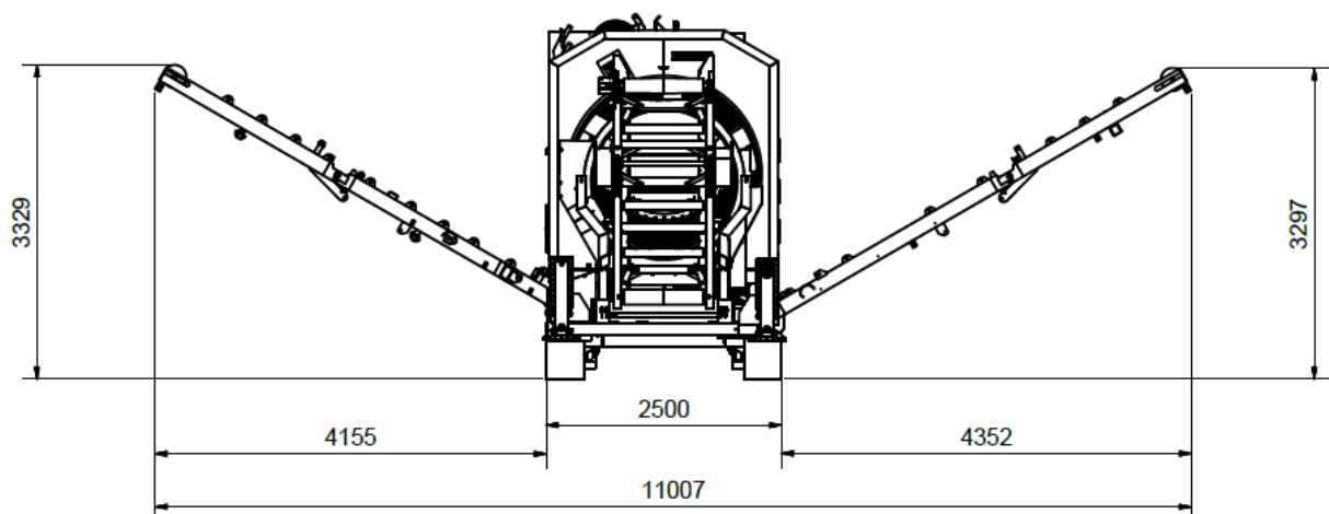
Fig. 12-2: Installation complète (vue de derrière)
