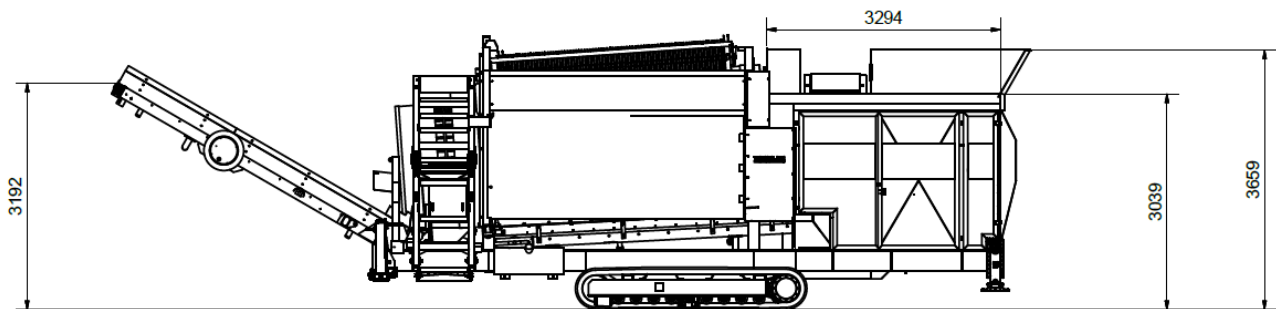
Fig. 12-1: Installation complète (remorque)
