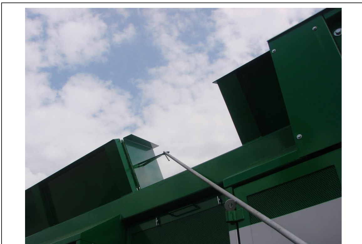
Fig. 8-5: Barre à crochet et boucle de la porte de service
