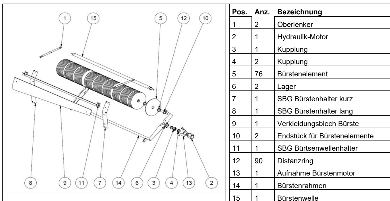
Fig. 11-7: Construction et montage des éléments de la brosse
