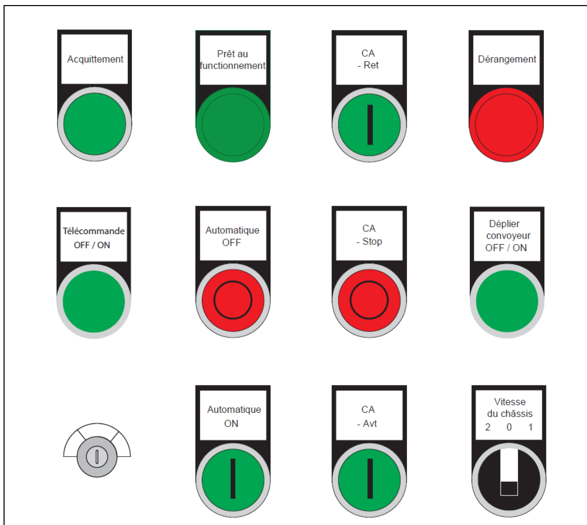
Fig. 4-3: Affichage de commande et d'état
