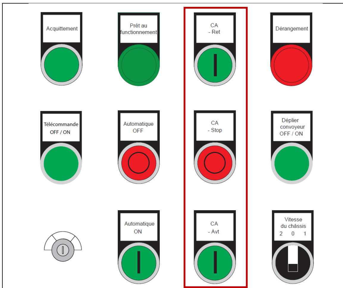
Fig. 8-6 : unité de commande
