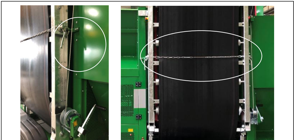
Fig. 7-2 : Sécurisation du transport de la 1. Fraction
