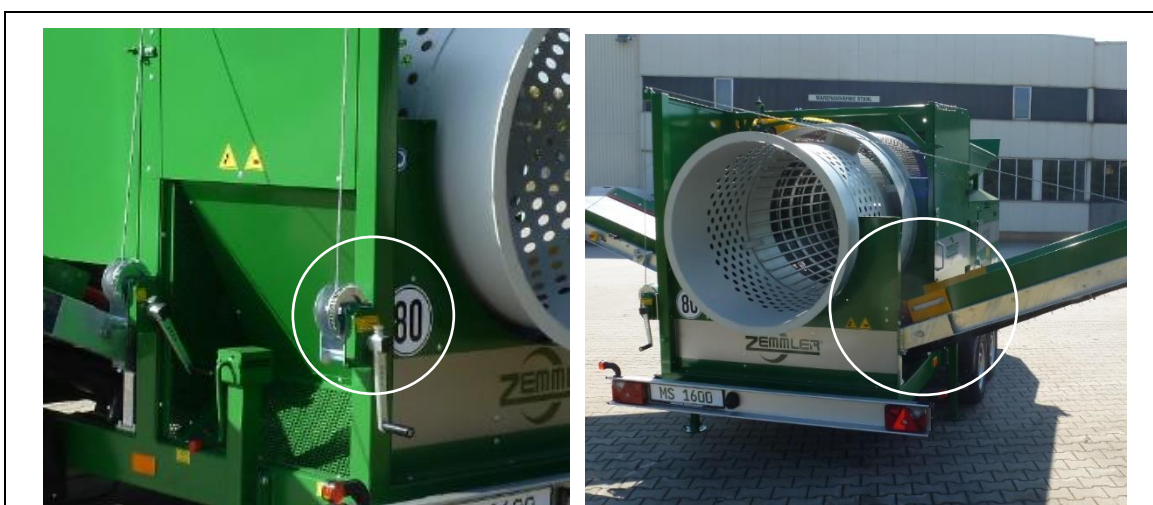
Fig. 8-2 : Treuil et tôles de guidage du 2ème tapis de fractionnement
