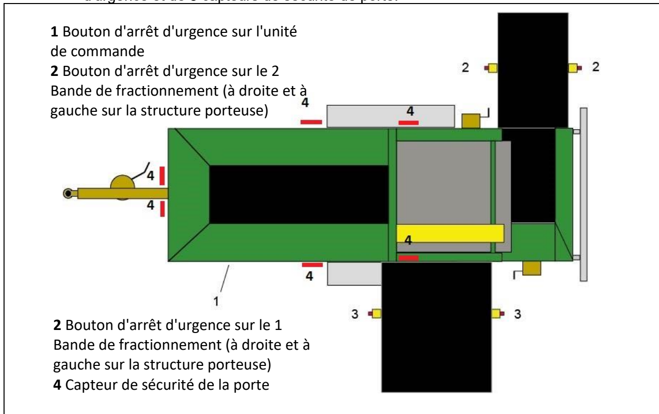
Fig. 3-1 : Position des dispositifs de sécurité
