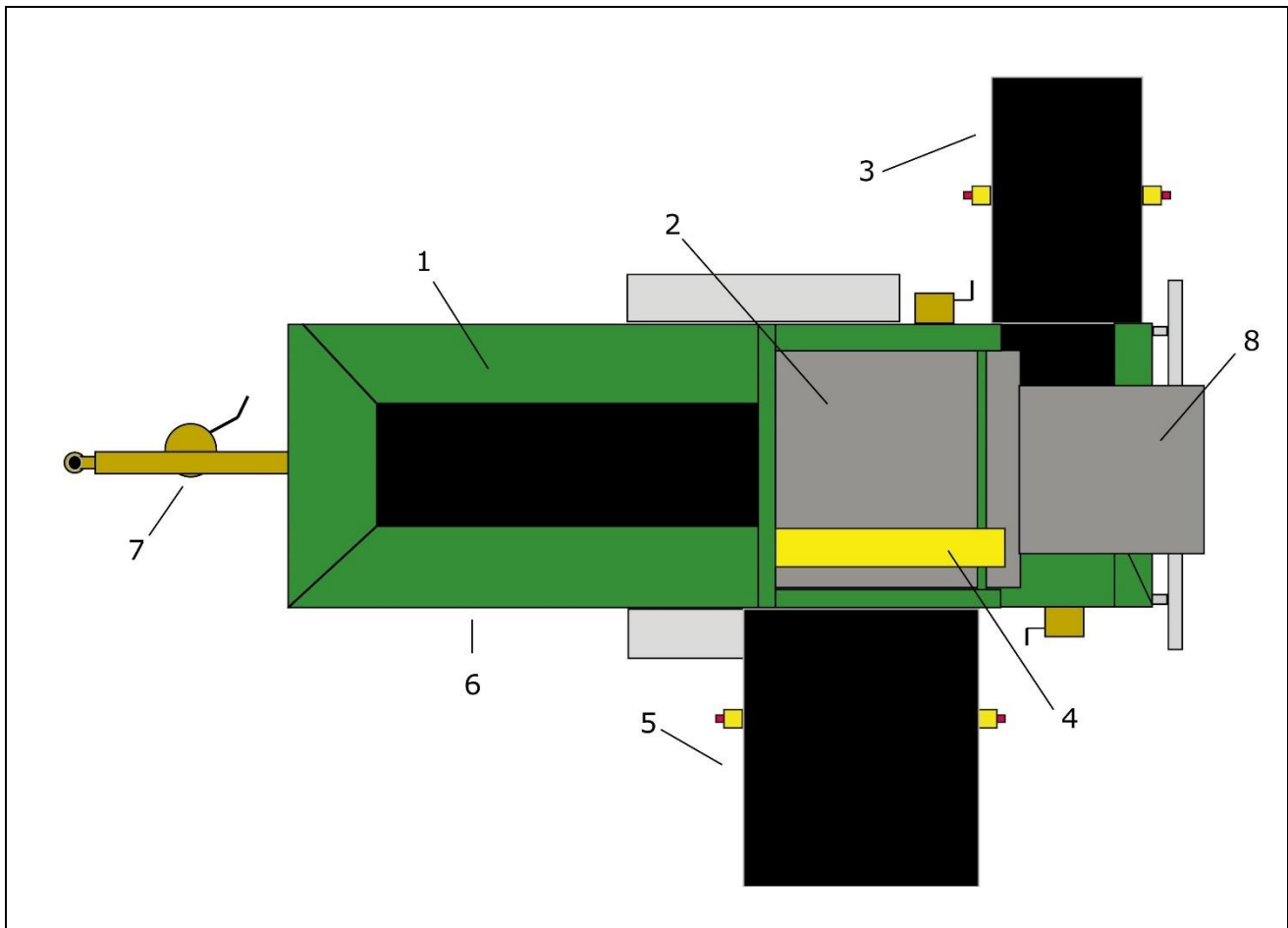
Fig. 4-1 : Aperçu des composants (vue de dessus)
