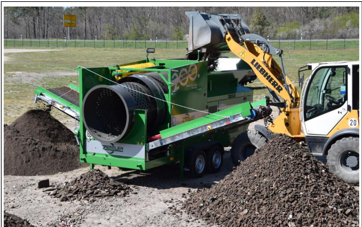
Fig. 6-1 : Exemple d'installation de criblage en position de travail (vue de l'avant gauche)
