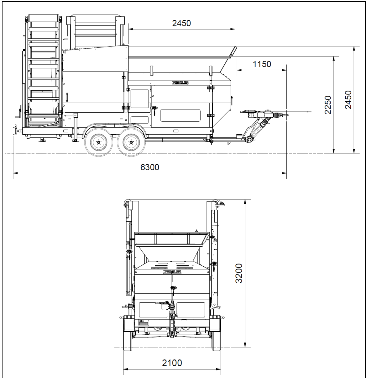
Fig. 12-1: Ensemble de l'installation Position de transport
