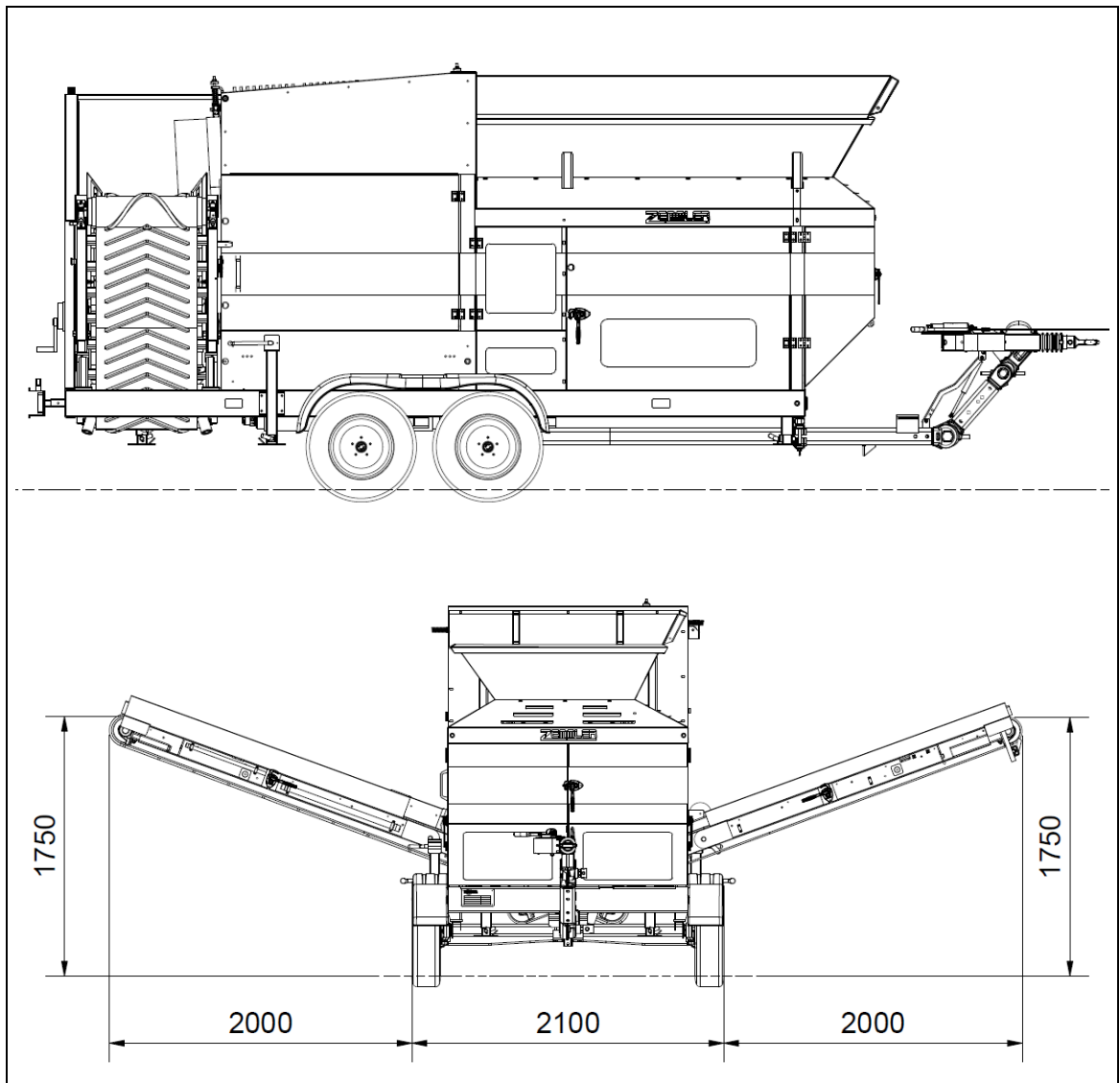
Fig. 12-2: Installation complète Position de travail
