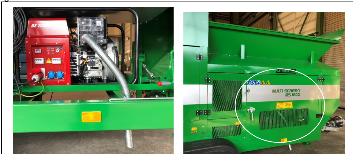
Fig. 8-3 Exemple de pose du tuyau d'échappement
