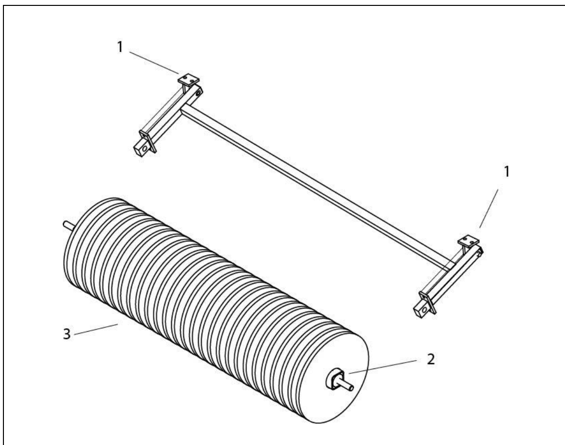
Fig. 11-6 : Structure et fixation de l'élément de brosse
