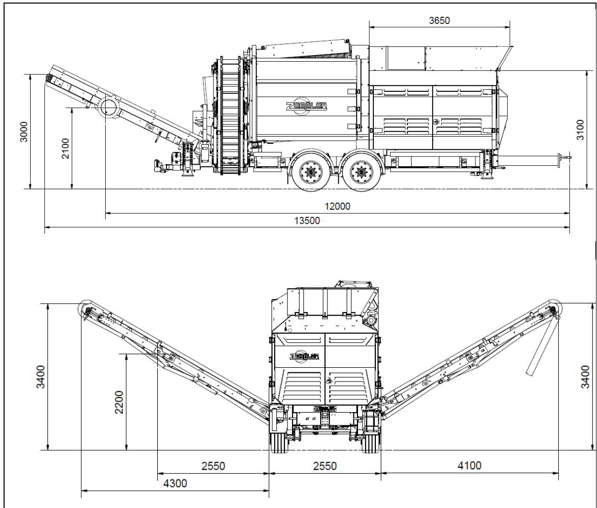
Obr. 12-2: Celková pracovní poloha stroje s opcí prodlouženého dopravníku pro střední a hrubou frakci
